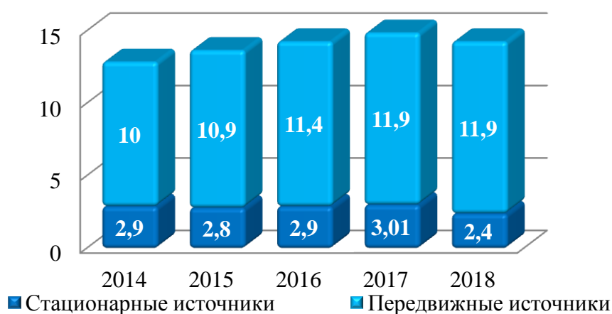
Динамика выбросов загрязняющих веществ в атмосферный воздух (тыс. тонн)
